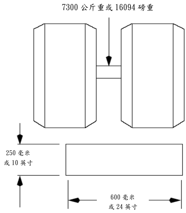
圖二二六～二 車輪荷重面積
