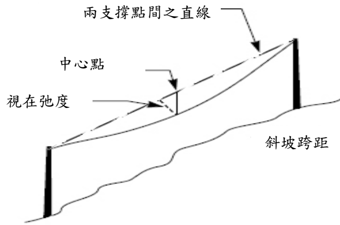
圖七 弛度及視在弛度
