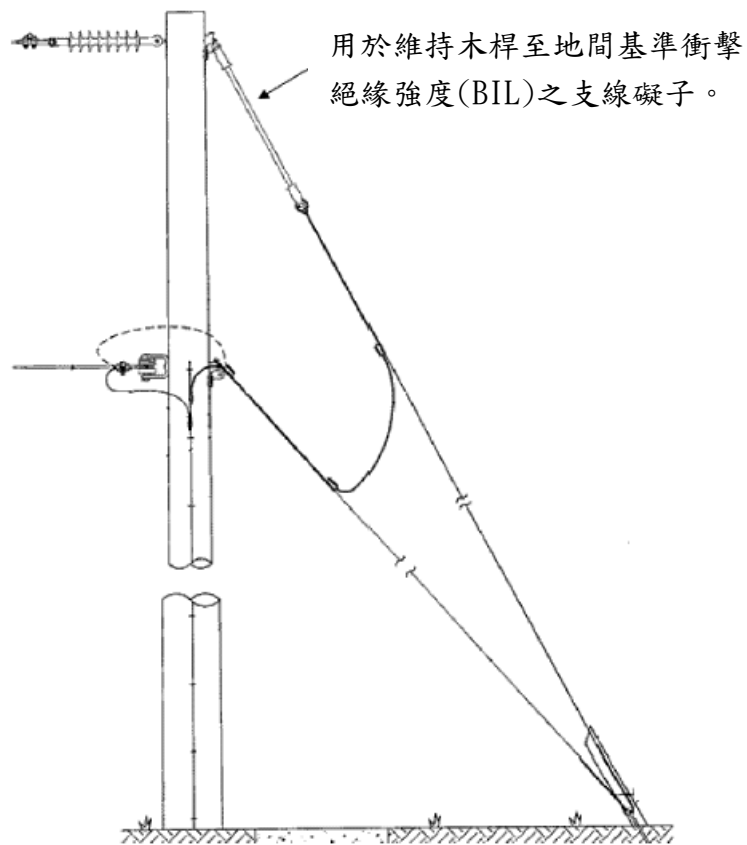
圖二一一 基準衝擊絕緣強度 (BIL) 絕緣之礙子
